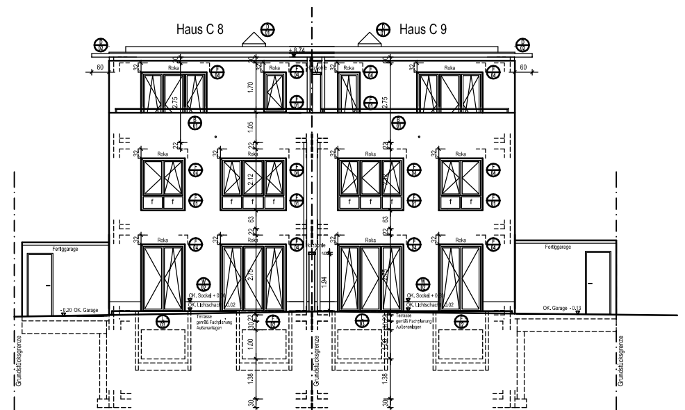
Ansicht Süd
