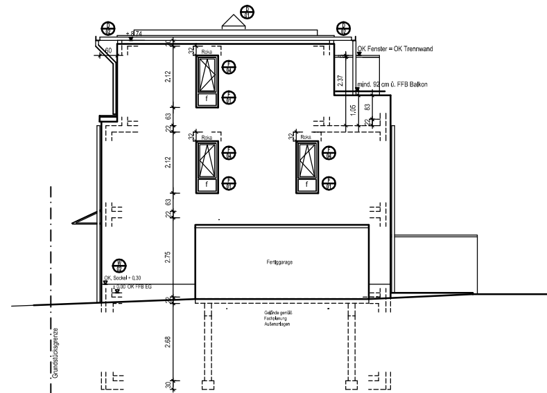
Ansicht West
