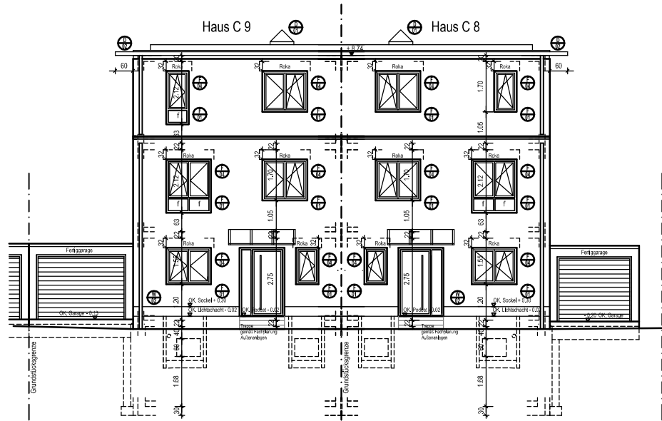
Ansicht Nord
